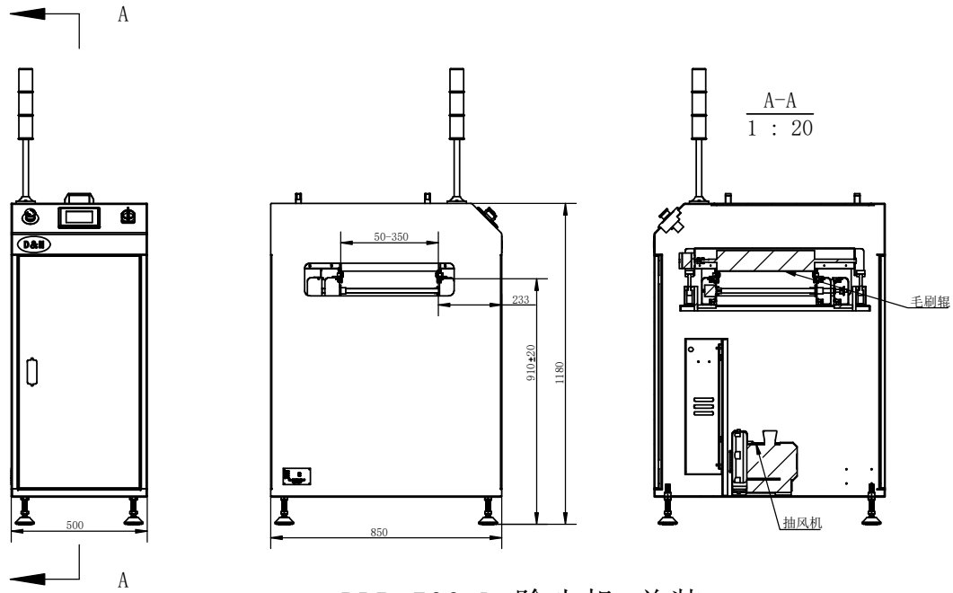
DDR-500-L-除尘机-总装
